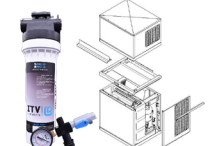
STACKING KIT KIT APILADO
