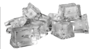
ALFA 14/19gr 36 mm (W) x 26 mm (D) x 23 mm (H) Average dimensions Dimensiones promedio
