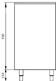
LEFT SIDE VIEW VISTA LATERALE SINISTRA
