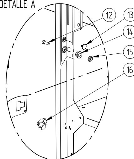
DETALLE A
